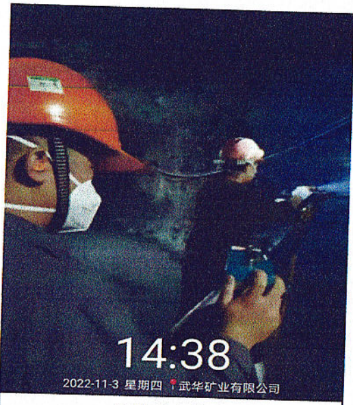
风钻粉尘检测
