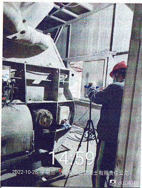
搅拌机粉尘检测 2022.10.26
