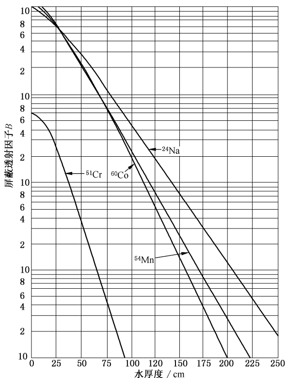
图 B.2 放射性核素屏蔽透射因子与水厚度的关系(引自 \gamma 射线屏蔽参数手册)
