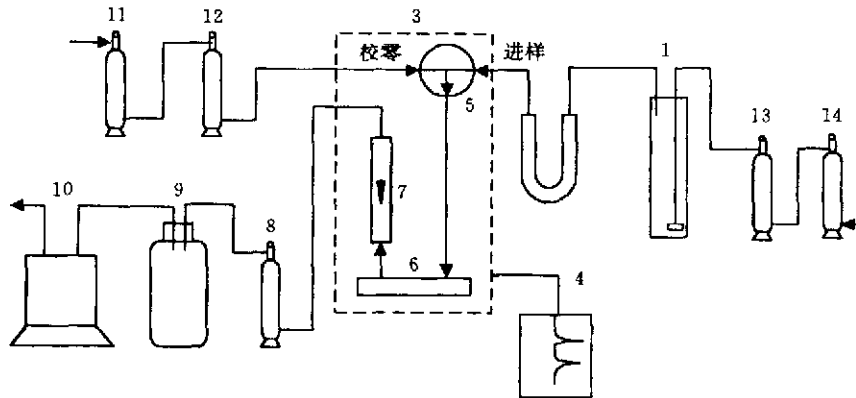
1—汞还原器; 2—U型管; 3—测汞仪; 4—记录仪; 5—三通阀; 6—吸收池; 7—流量控制器; 8、12、13—汞吸收塔; 9—气体缓冲瓶; 10L、10—机械真空泵; 11、14—空气干燥塔(内盛变色硅胶)
