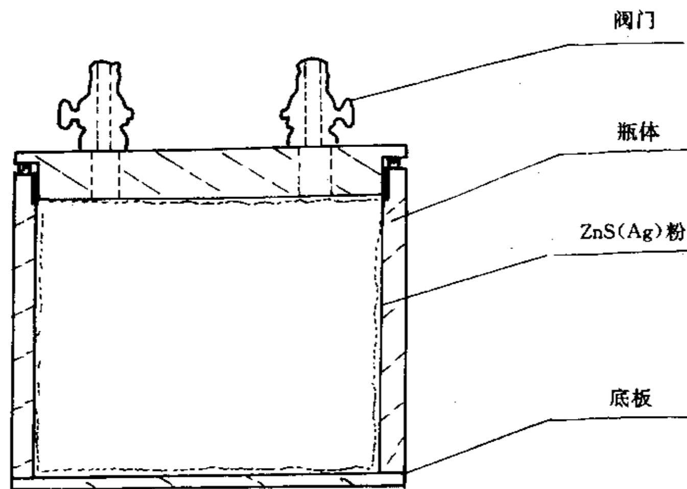
图1 闪烁瓶简图
