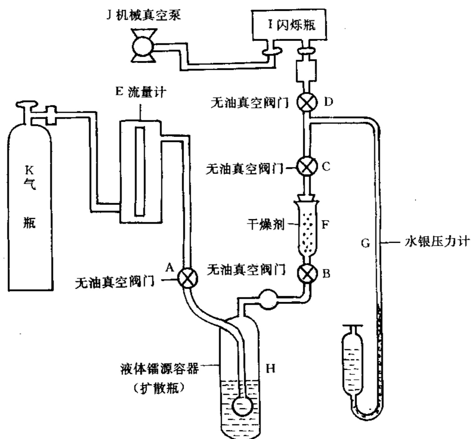
图2 玻璃刻度系统示意图
