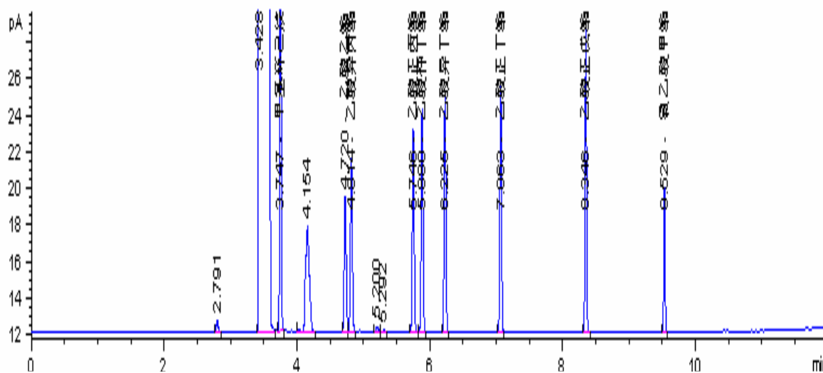
图1 色谱分离图
